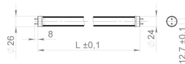
Рис. 1. Габаритные размеры светильника.
