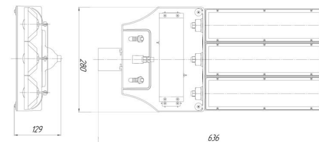
Рис. 1. Габаритные размеры светильника.
