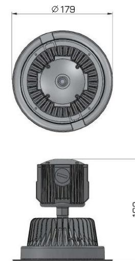
Рис. 1. Габаритные размеры светильника
