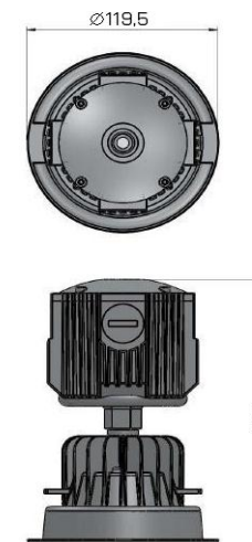
Рис. 1. Габаритные размеры светильника
