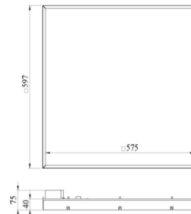
Рис. 1. Габаритные размеры светильника
